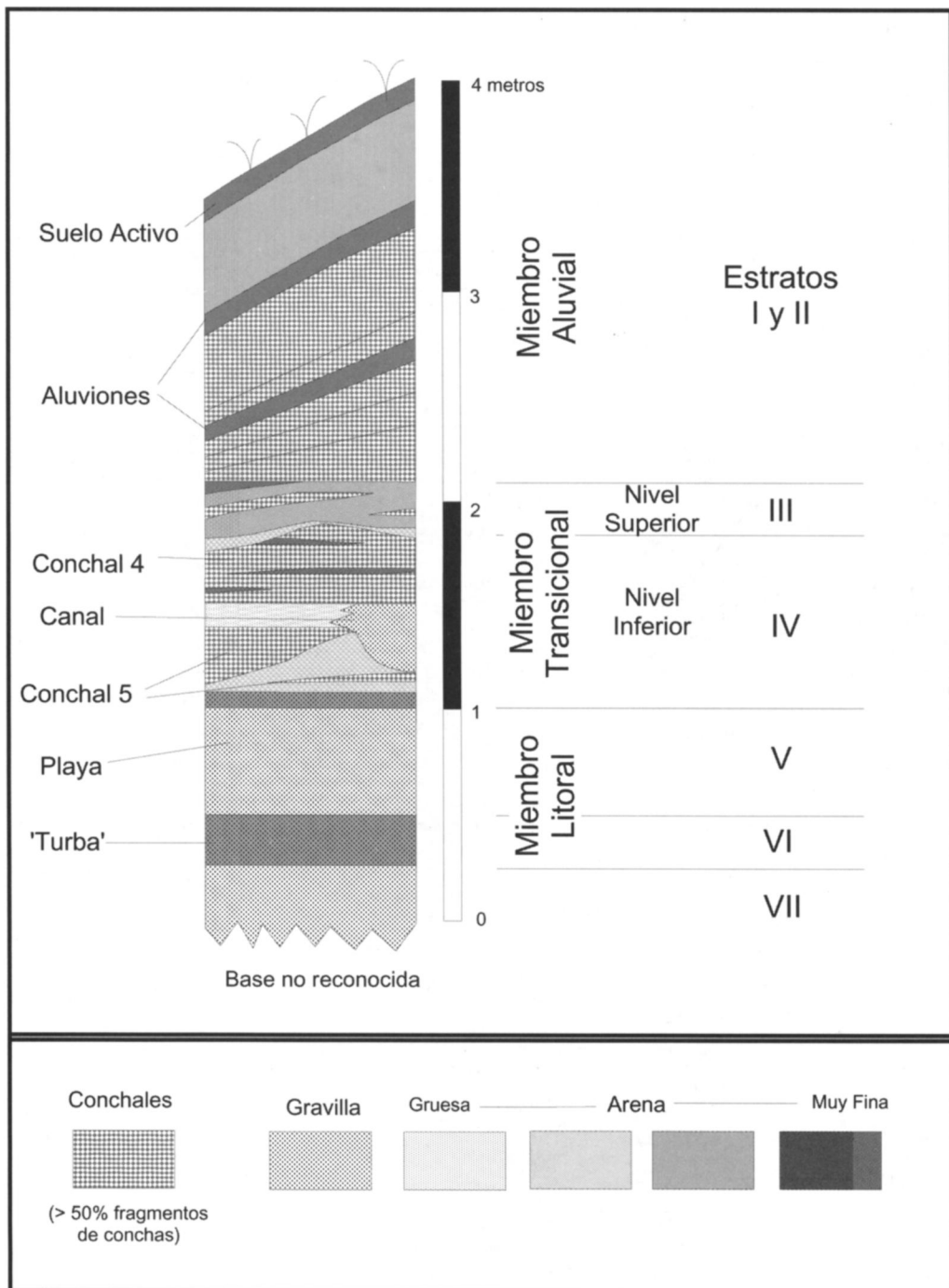
Figura 1. Columna estratigráfica sitio Piedra Azul.
