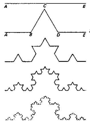
La curva de Von Koch: ¡más que una línea, menos que una superficie! Al segmento AE (1) se le quita su segundo tercio y se sustituye por el triángulo BCD (2). En (3), se repite esta operación con cada uno de los segmentos AB, BC, CD y DE separadamente. Se obtiene así un trazado anguloso en el que todos los segmentos son iguales. En cada uno de estos segmentos se repite por tercera vez (4) la operación anterior (2) y (3); y así sucesivamente, hasta el infinito. De ese modo, en el límite se obtiene una "curva" formada por un número infinito de puntos angulosos y que no admite tangente en ninguno de sus puntos. La longitud de esa curva es infinita y su dimensión es superior a uno: representa un espacio de dimensión 1,261\ 859 (exactamente \log 4/\log 3 ).
