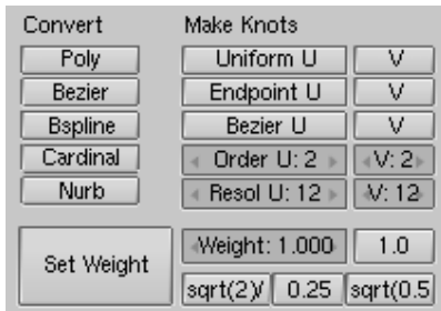
Pesos preconfigurados
