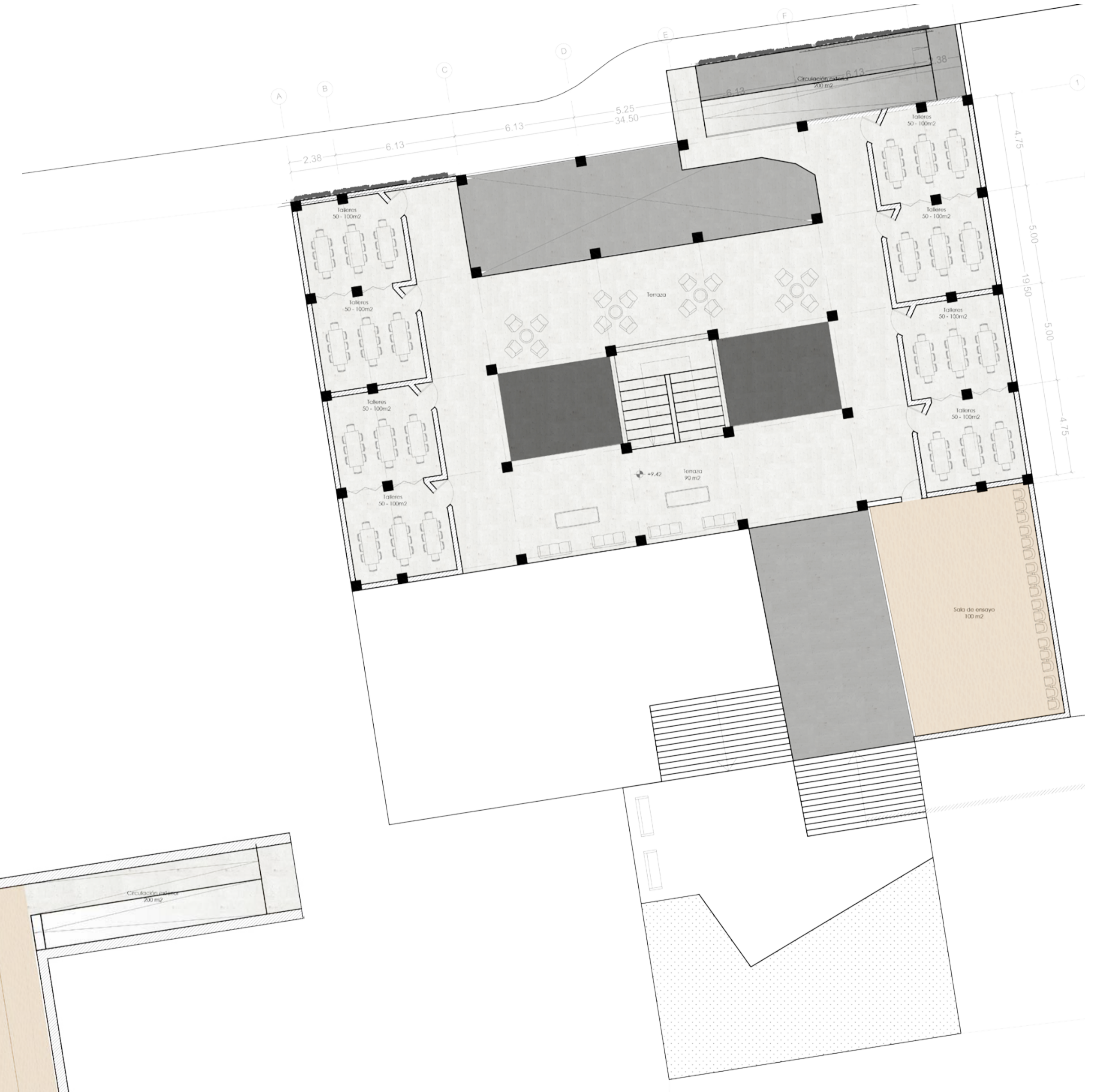
Planta nivel 4
