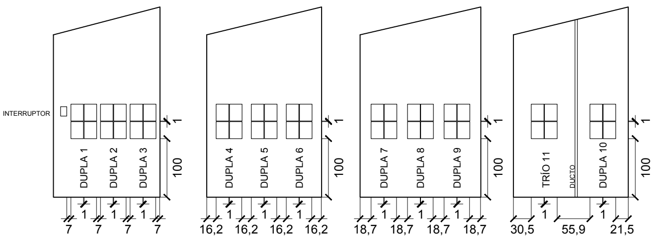
MURO A
