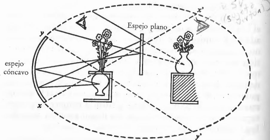
Esquema simplificado de los dos espejos
