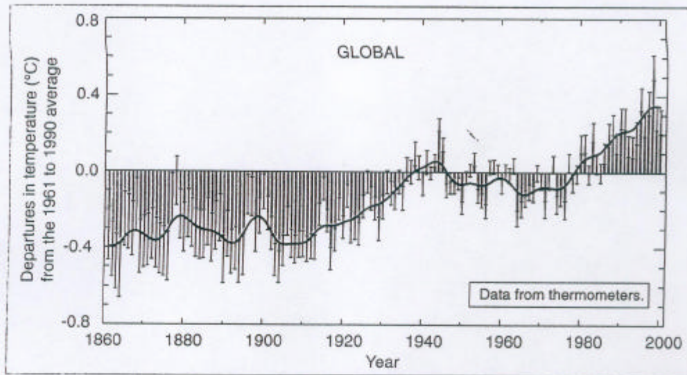
Anomalías anuales combinadas de la temperatura superficial (tierra y mar) respecto del promedio entre 1961-1990. Barras representan incertidumbre (errores estándar).
