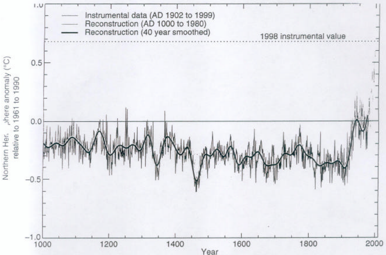
Reconstrucción de anomalías de temperatura para el hemisferio norte entre 1000 y 1980 (línea delgada) y valor suavizado con filtro de 40 años (línea gruesa). Con fines de comparación se indica el valor instrumental para 1998.
