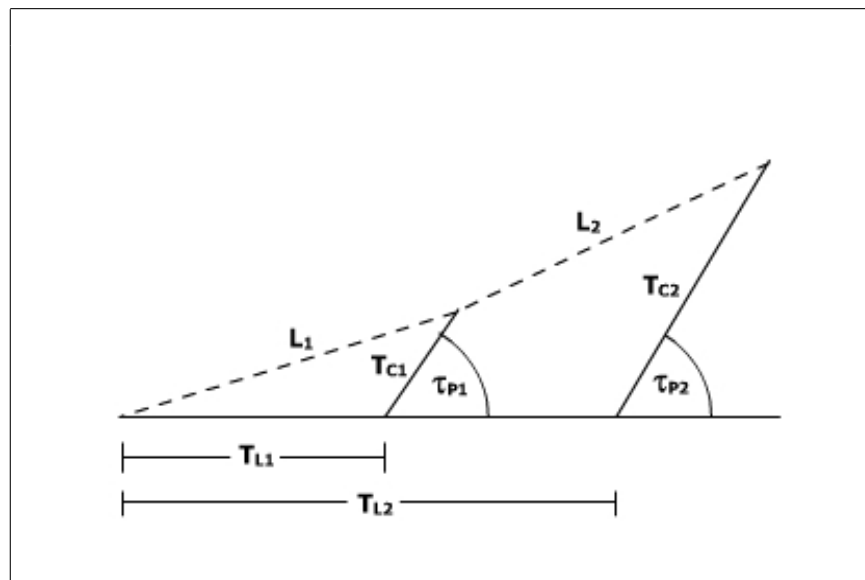
Figura 2.23: Clotoide replanteada
