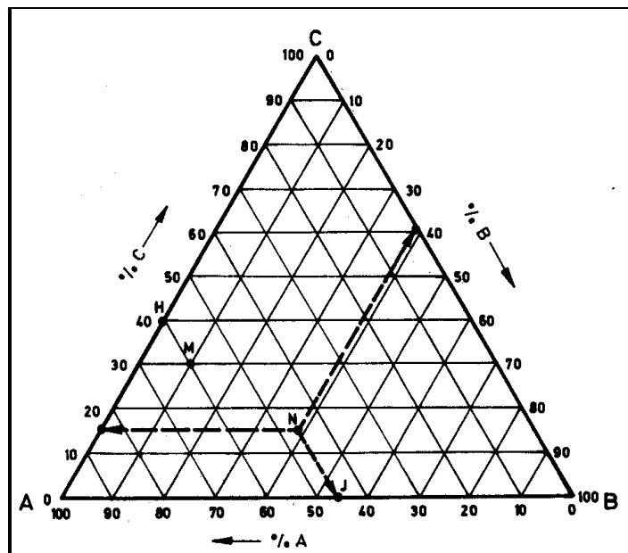
Figura 8.1 Diagrama Triangular para Mezclas Ternarias (Tomado de Custodio; Llamas, 1976)
