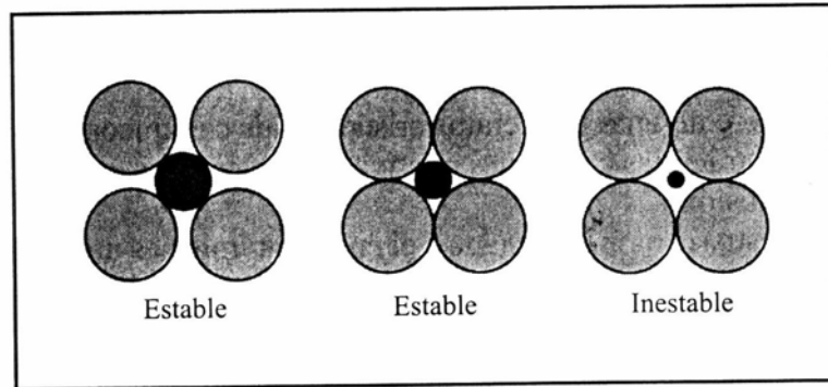
Figura 1. Esquema bidimensional del efecto de los tamaños relativos de los iones de un cristal iónico (factor geométrico), sobre la estabilidad del cristal. Para que la situación sea geoméricamente estable, el catión debe estar en contacto con los aniones de su entorno.
