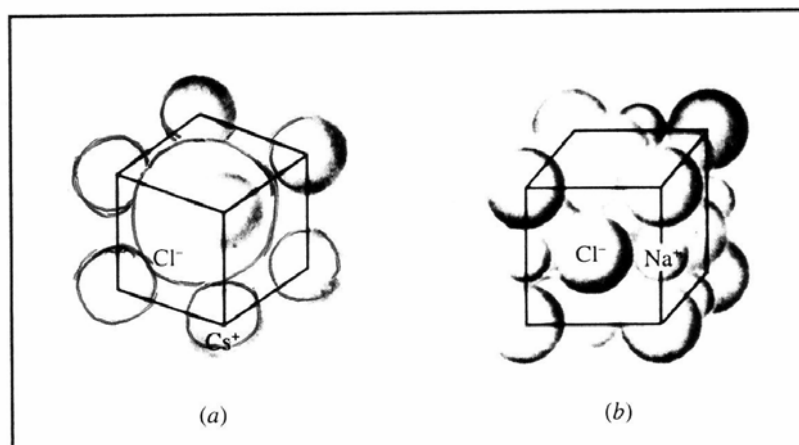
Figura 2.13. Disposiciones de empaquetamiento iónico en (a) \text{CsCl} y (b) \text{NaCl} . Ocho iones \text{Cl}^- se pueden empaquetar en torno a un ion \text{Cs}^+ , pero sólo seis iones \text{Cl}^- se pueden empaquetar en torno a un ion \text{Na}^+ .
