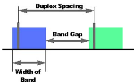
Ilustración 2: Explicación tecnología FDD
