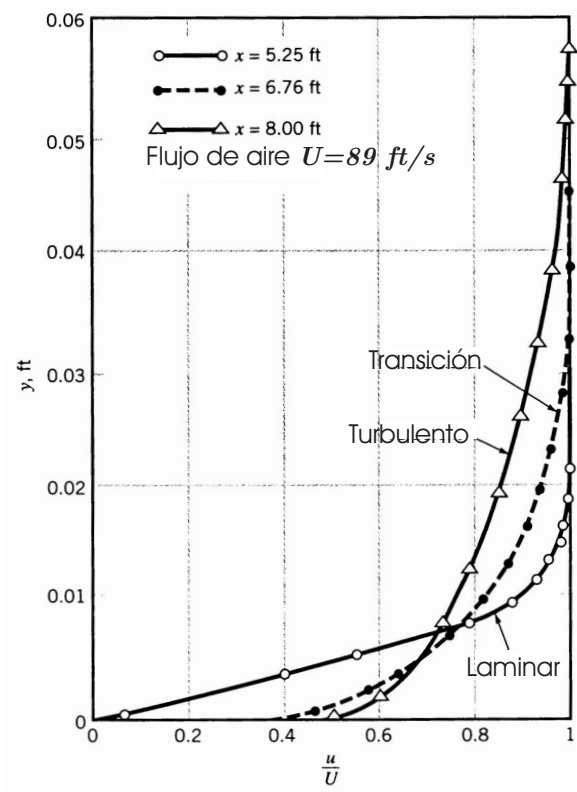
Figura 10.15: Variación típicas del perfil de velocidades para distintos tipos de regímenes.
