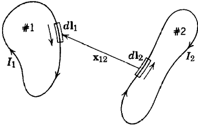
Fig. 5.3 Two Ampèrian current loops.
