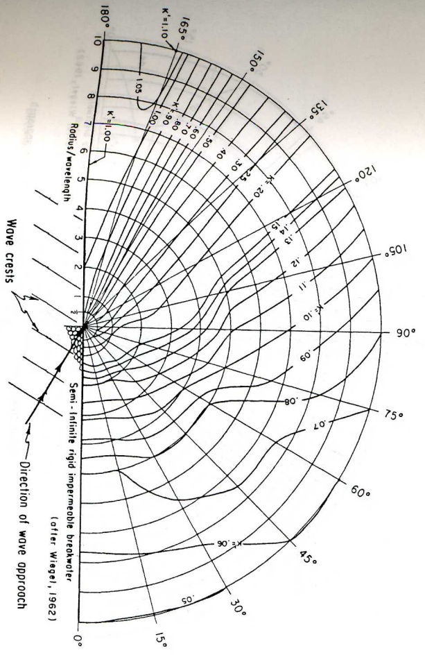
Figura 1.54 Diagrama de difracción. Ángulo de incidencia 150°
