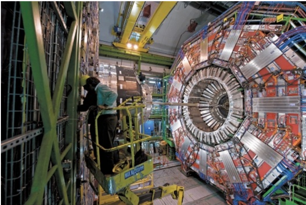
El detector CMS en construcción. © CERN
