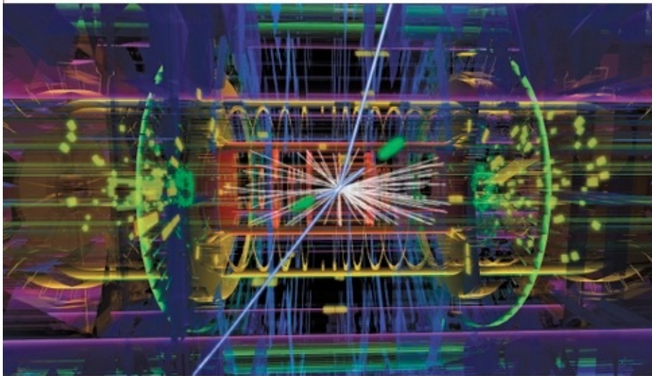
Un posible evento Higgs en el detector ATLAS. Las dos largas líneas azules son muones, y las líneas azules cortas son electrones, de manera que esto podría representar la desintegración del Higgs en dos bosones Z. © CERN
