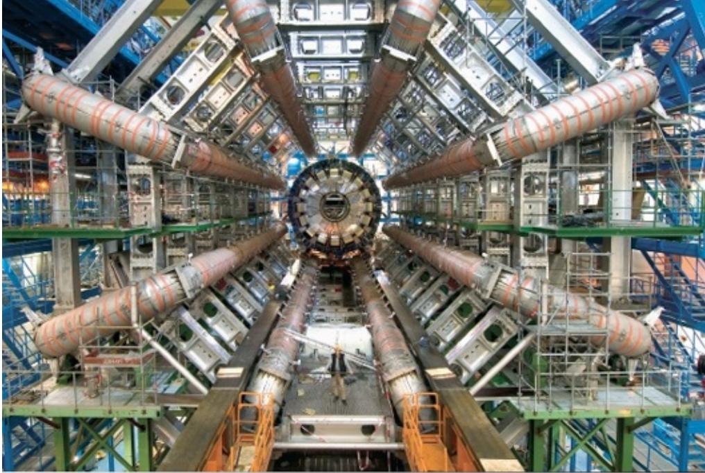
El detector ATLAS en construcción. Fijese en la persona que aparece en la zona inferior del centro de la imagen. Las ocho tuberías gigantes son imanes, que se utilizan para desviar a los muones y así poder medir sus energías. © CERN
