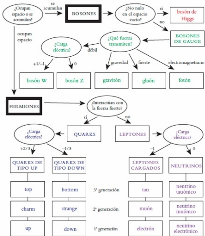
Diagrama de flujo que ilustra las partículas elementales del Modelo Estándar. Esta es la versión moderna de la tabla periódica de los elementos. Los quarks aparecen en azul, los leptones en morado, los bosones de gauge en verde y el bosón de Higgs en rojo. SEAN CARROLL
