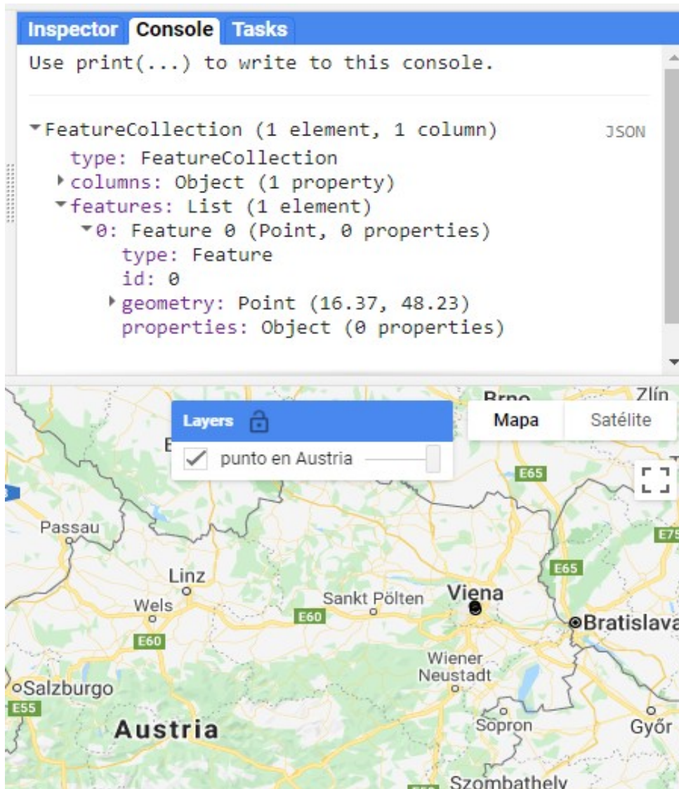
Figura 8.3: Visualización de una colección de vectores con un único objeto de geometría de tipo punto.
