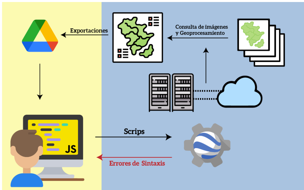
Figura 5.1: Representación de los dos lados de programación en GEE: del cliente (amarillo) y el servidor (azul).
