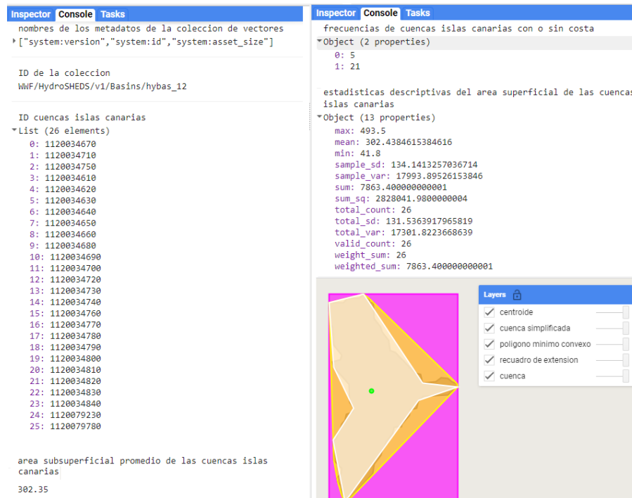
Figura 8.8: Ejemplos de la salida en la consola de diferentes propiedades de los vectores que forman una colección de vectores de cuencas.
