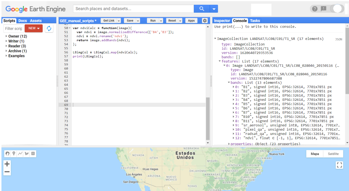
Figura 10.19: Consulta de información en la consola para verificar que la colección de imágenes contiene la banda NDVI.
