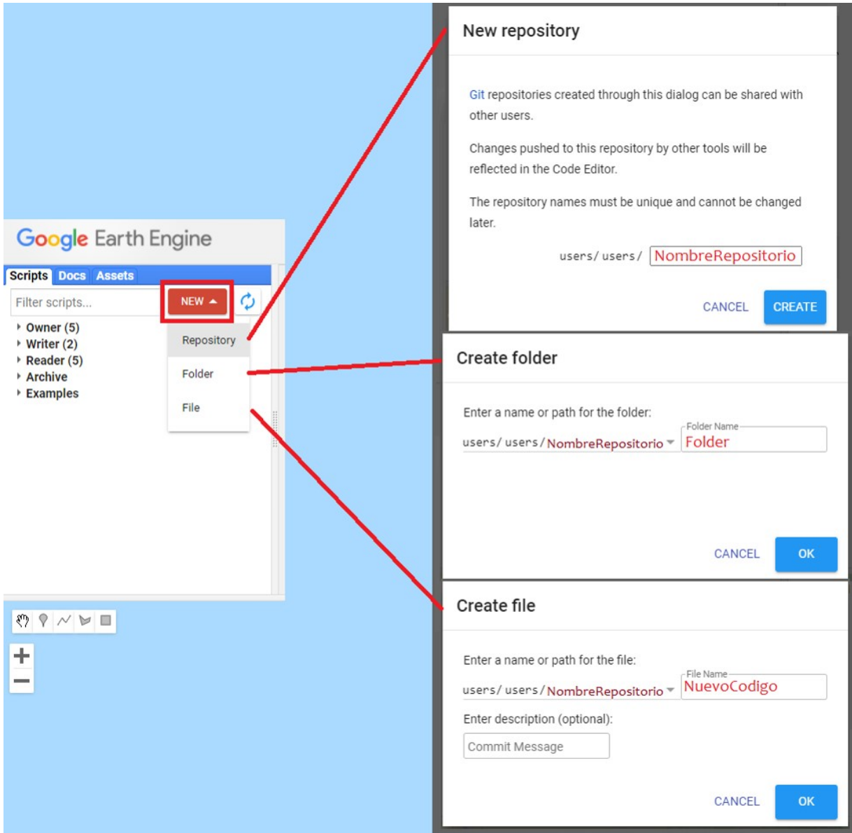
Figura 2.5: Opciones disponibles dentro de la pestaña de Nuevo.
