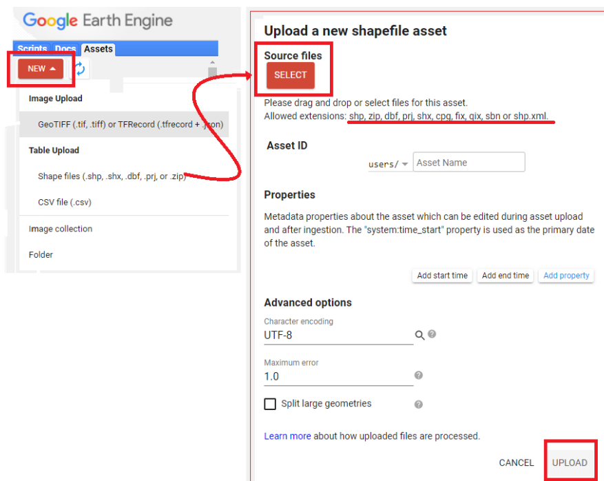
Figura 4.1c: Opciones disponibles para importar datos tipo Shapefile, incluir todos los archivos auxiliares.
