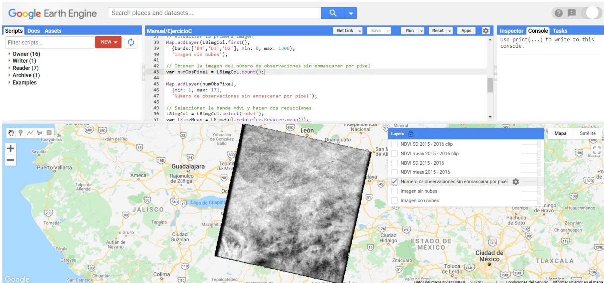
Figura 10.21: Visualización de la imagen con el número de observaciones sin enmascarar por píxel.
