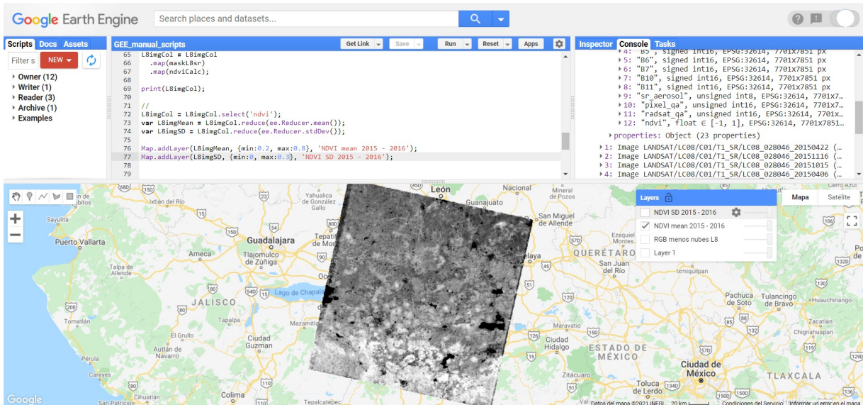
Figura 10.20: Visualización de la imagen de NDVI promedio.
