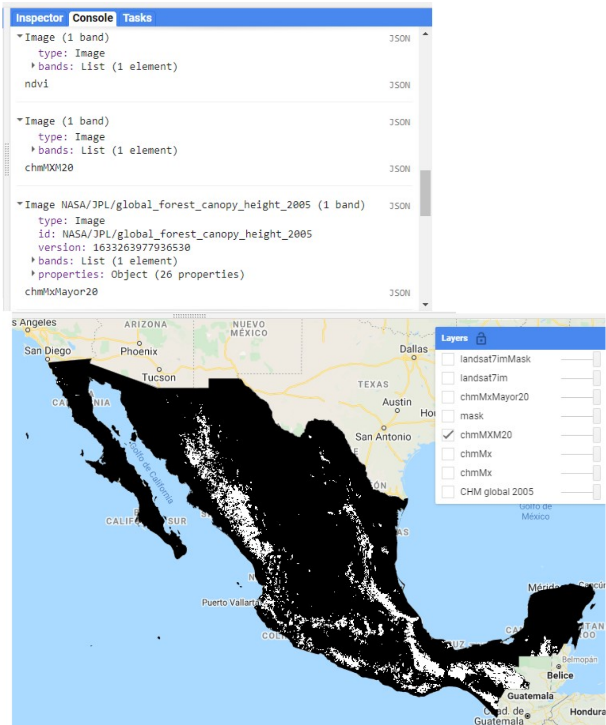
Figura 9.7: Resultado de la máscara booleana de altura del dosel.
