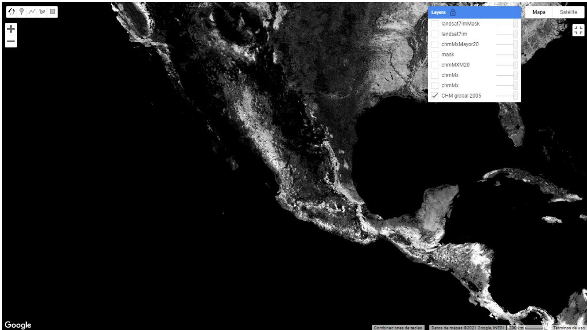
Figura 9.4: Visualización de la capa de la altura del dosel
