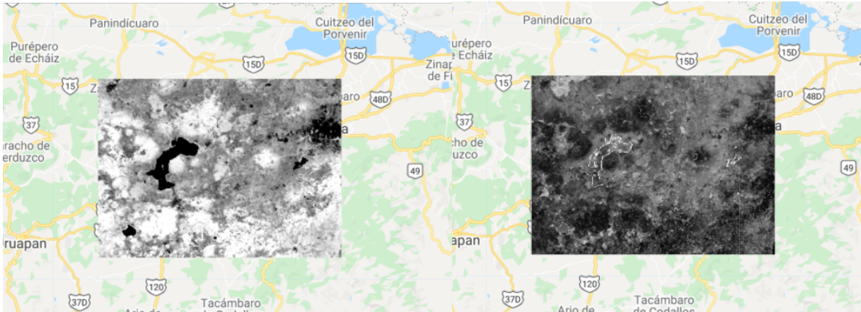
Figura 10.22: Visualización de los compuestos de media y desviación estándar cortados.
