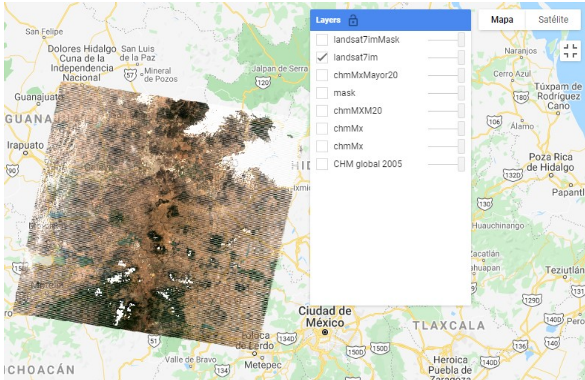
Figura 9.10: Imagen Landsat antes del enmascaramiento de nubes.
