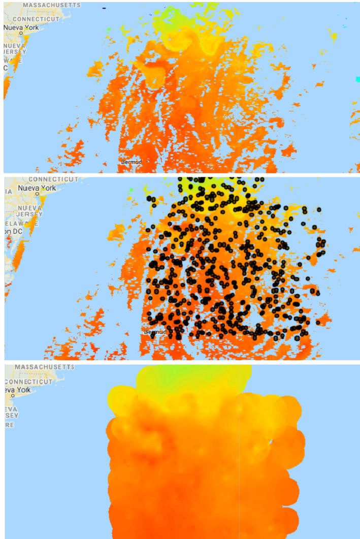
Figura 11.4: Visualización de la capa inicial de temperatura de la superficie marina (superior), puntos de muestreo (medio) y capa interpolada (inferior).
