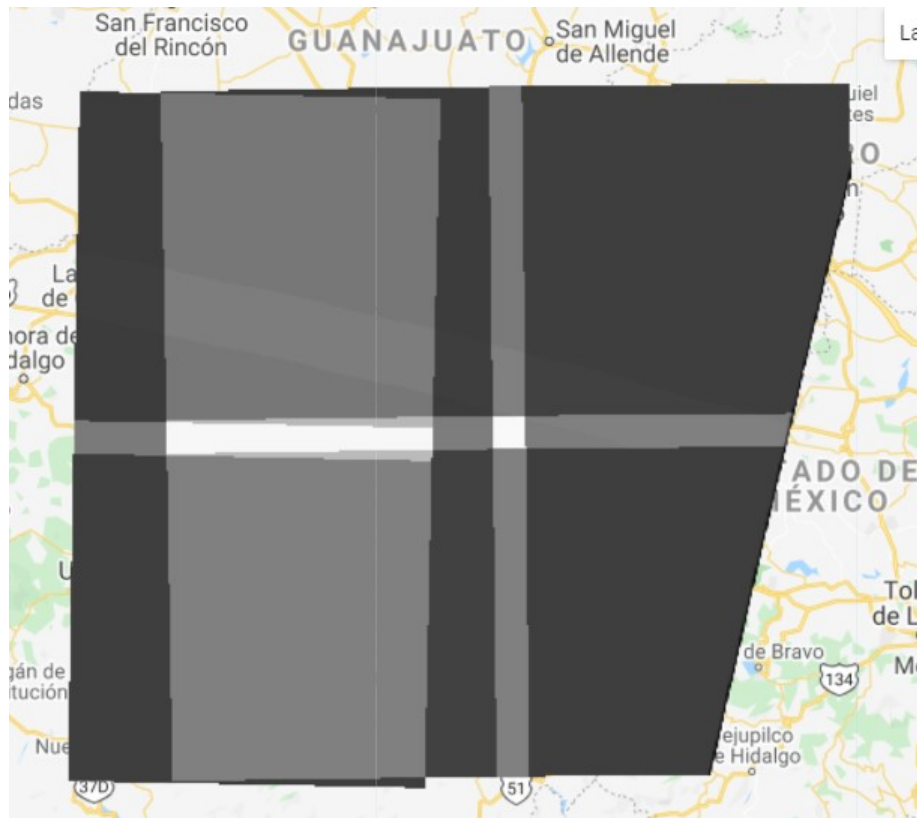
Figura 10.9: Visualización de la imagen del conteo de observaciones.
