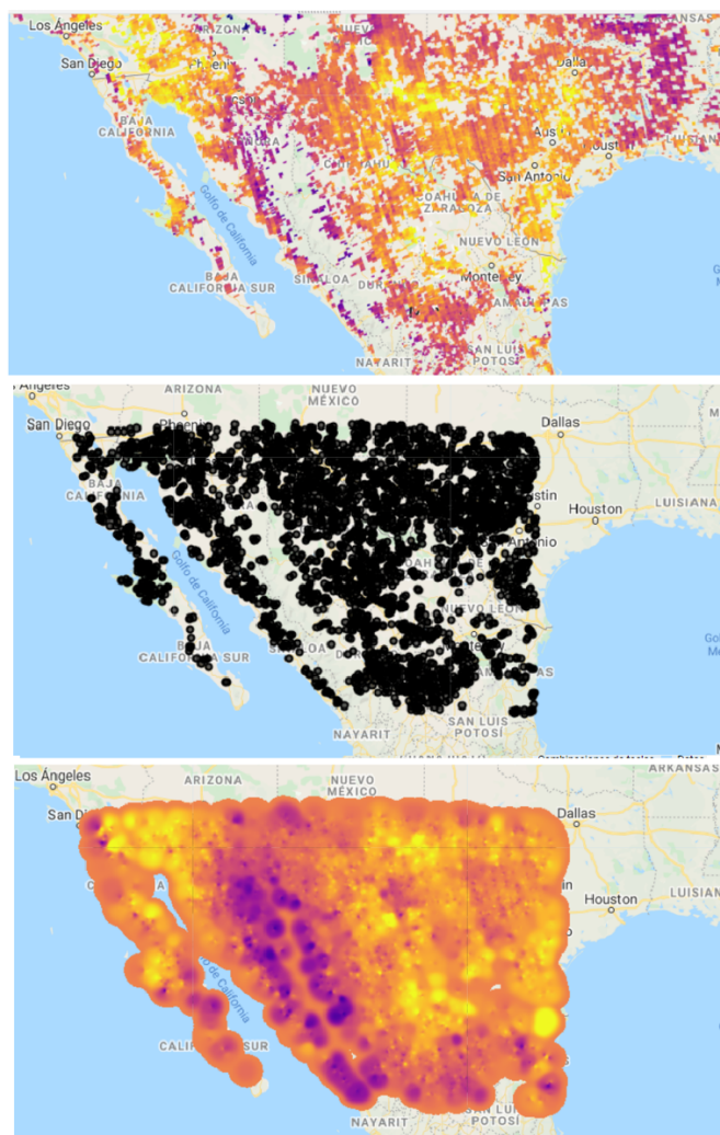
Figura 11.3: Visualización de la capa inicial de CH_4 , (superior), puntos de muestreo (medio) e imagen interpolada (inferior).
