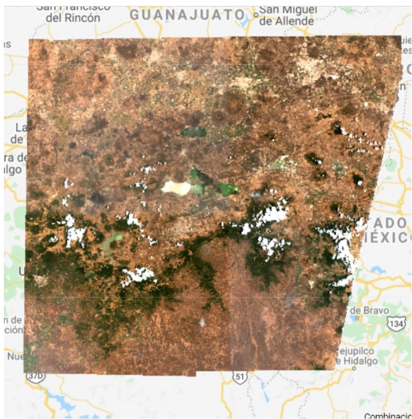
Figura 10.3: Visualización de la colección de imágenes de Sentinel-2 2A.
