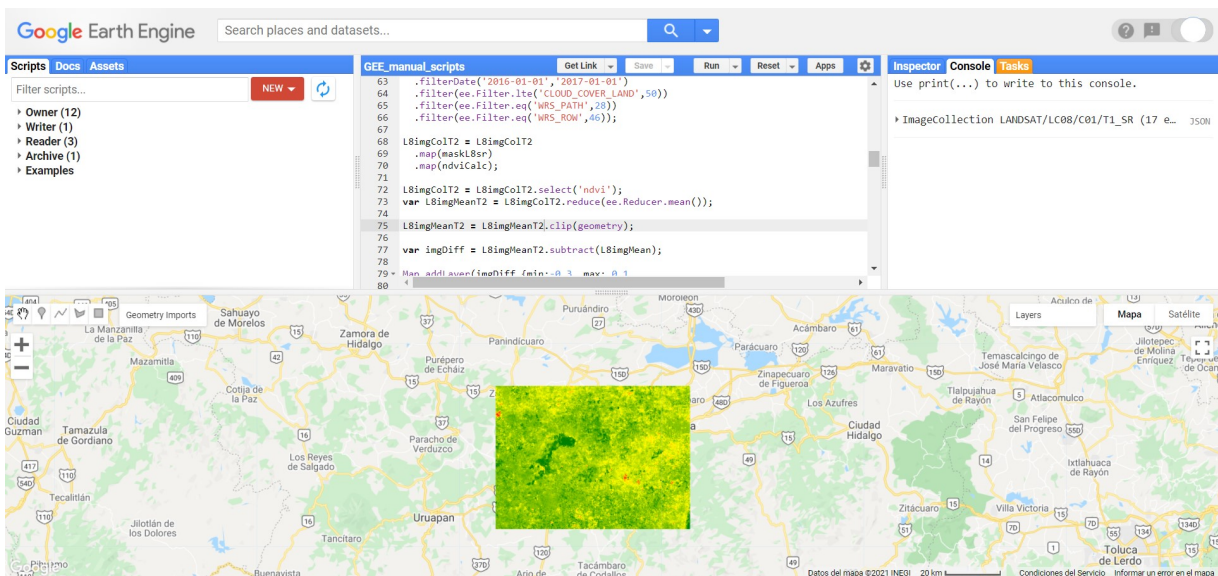
Figura 10.23: Imagen de la diferencia de NDVI entre dos años.
