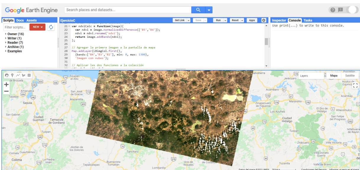
Figura 10.17: Ejemplo de una imagen con nubes.
