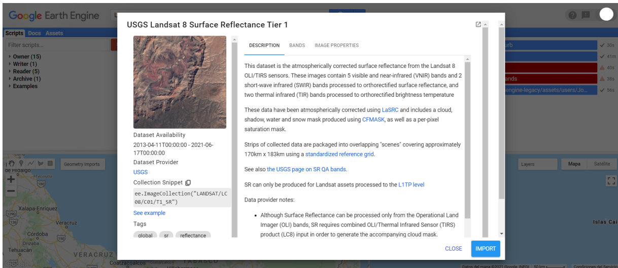
Figura 10.14: Consulta de propiedades de las imágenes contenidas en una colección de imágenes.
