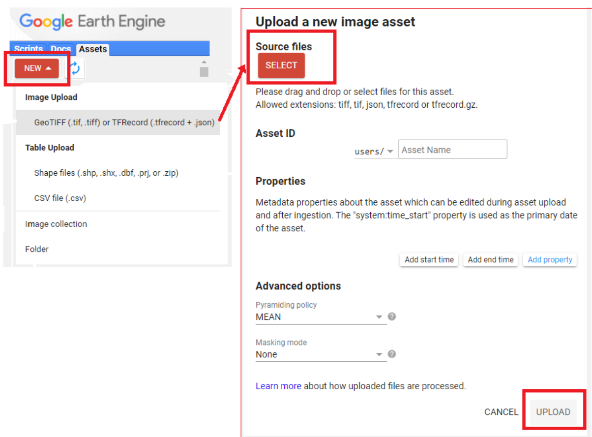
Figura 4.1a: Opciones disponibles para importar datos tipo raster (GeoTIFF o TFRecord).
