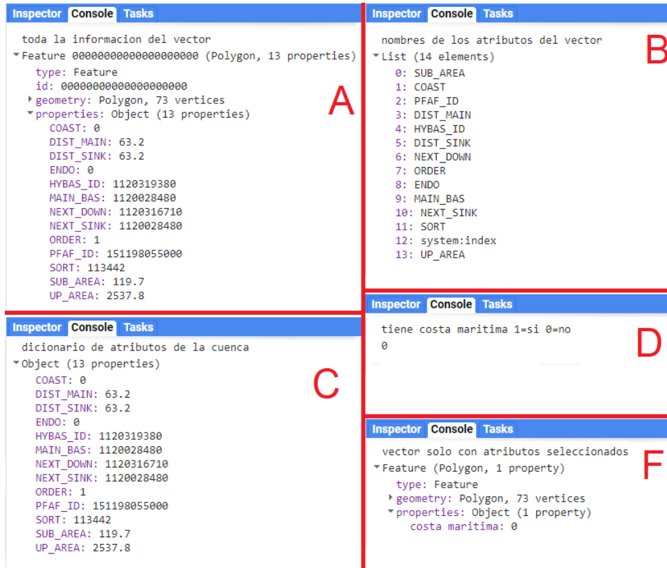
Figura 7.2: Salida de la consola de las propiedades (ejercicio 11) del vector "cuenca" (A), nombre de las propiedades de "cuenca" (B), propiedades como diccionario (C), valor del atributo "COAST" (D), renombrar el atributo (F)
