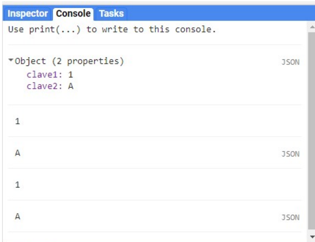
Figura 5.5: Salida de la consola de varios objetos de tipo diccionario.
