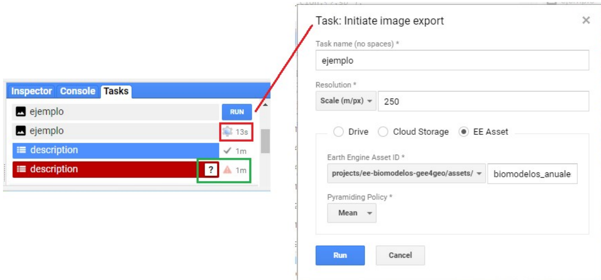
Figura 2.21: Vista de la pestaña de tareas dentro de GEE.
