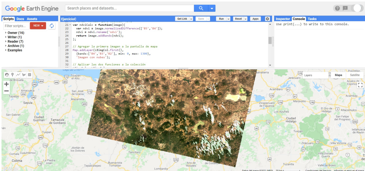
Figura 10.18: Ejemplo de una imagen donde se enmascararon las nubes.
