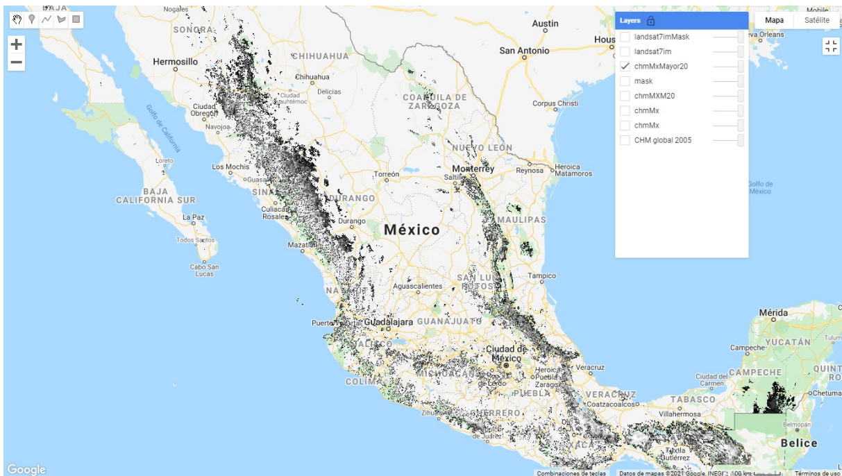
Figura 9.9: Resultado del enmascaramiento de la capa de altura del dosel.
