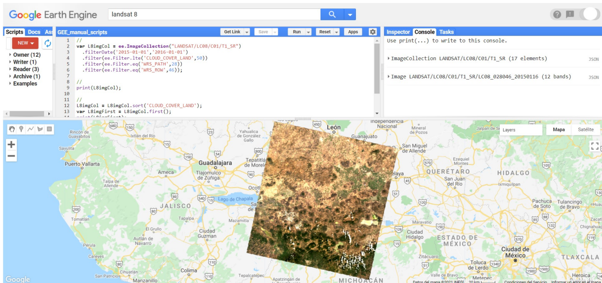
Figura 10.16: Visualización de la primera imagen de la colección de imágenes.
