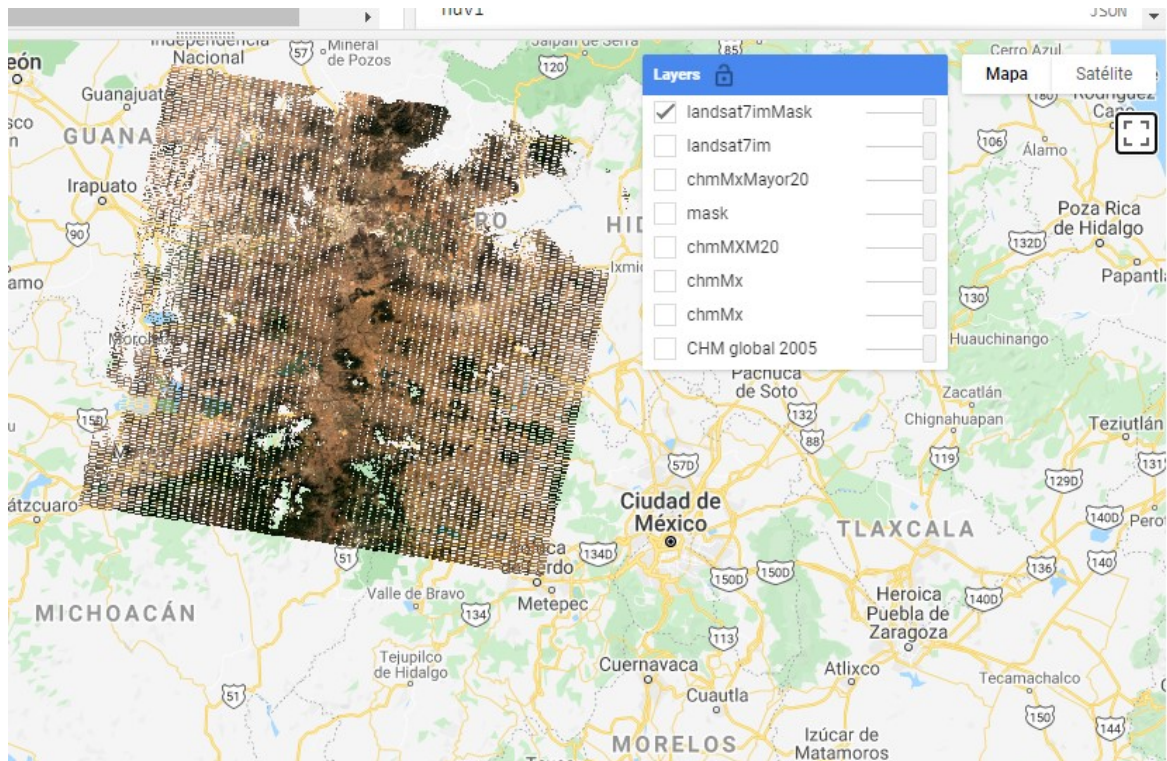
Figura 9.11: Imagen Landsat después del enmascaramiento de nubes. Nótese que las áreas enmascaradas ahora son transparentes.
