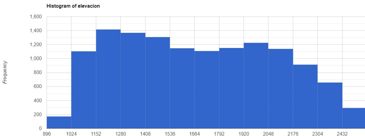
Figura 9.16: Histograma de valores del DEM.
