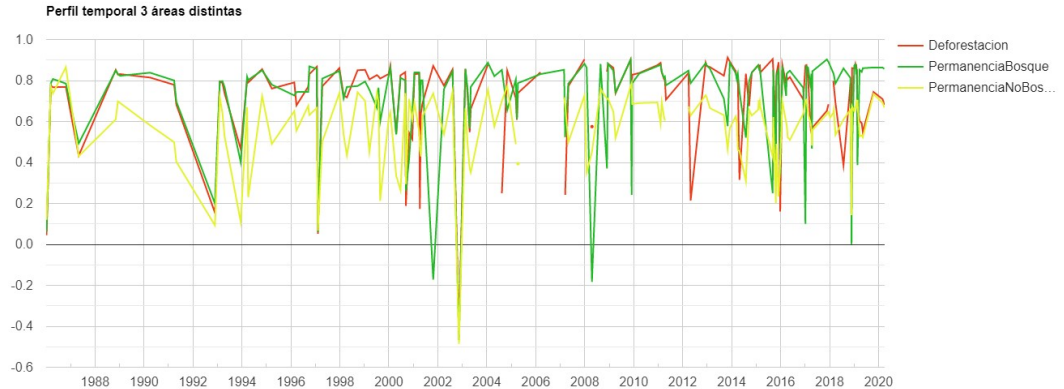
Figura 3.4: Ejemplo de un gráfico que muestra los perfiles temporales de un índice de vegetación (NDVI) en tres tipos de áreas: deforestación, permanencia de bosque y permanencia de no bosque.
