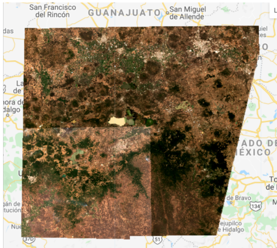
Figura 10.6: Visualización de la primera imagen de la colección.
