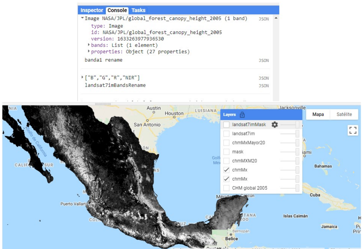
Figura 9.6: Visualización de la capa de altura del dosel en México.
