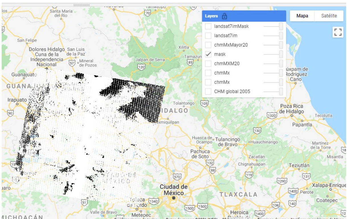
Figura 9.8: Visualización de la máscara de Landsat 8 indicando píxeles con nubes y sin nubes.
