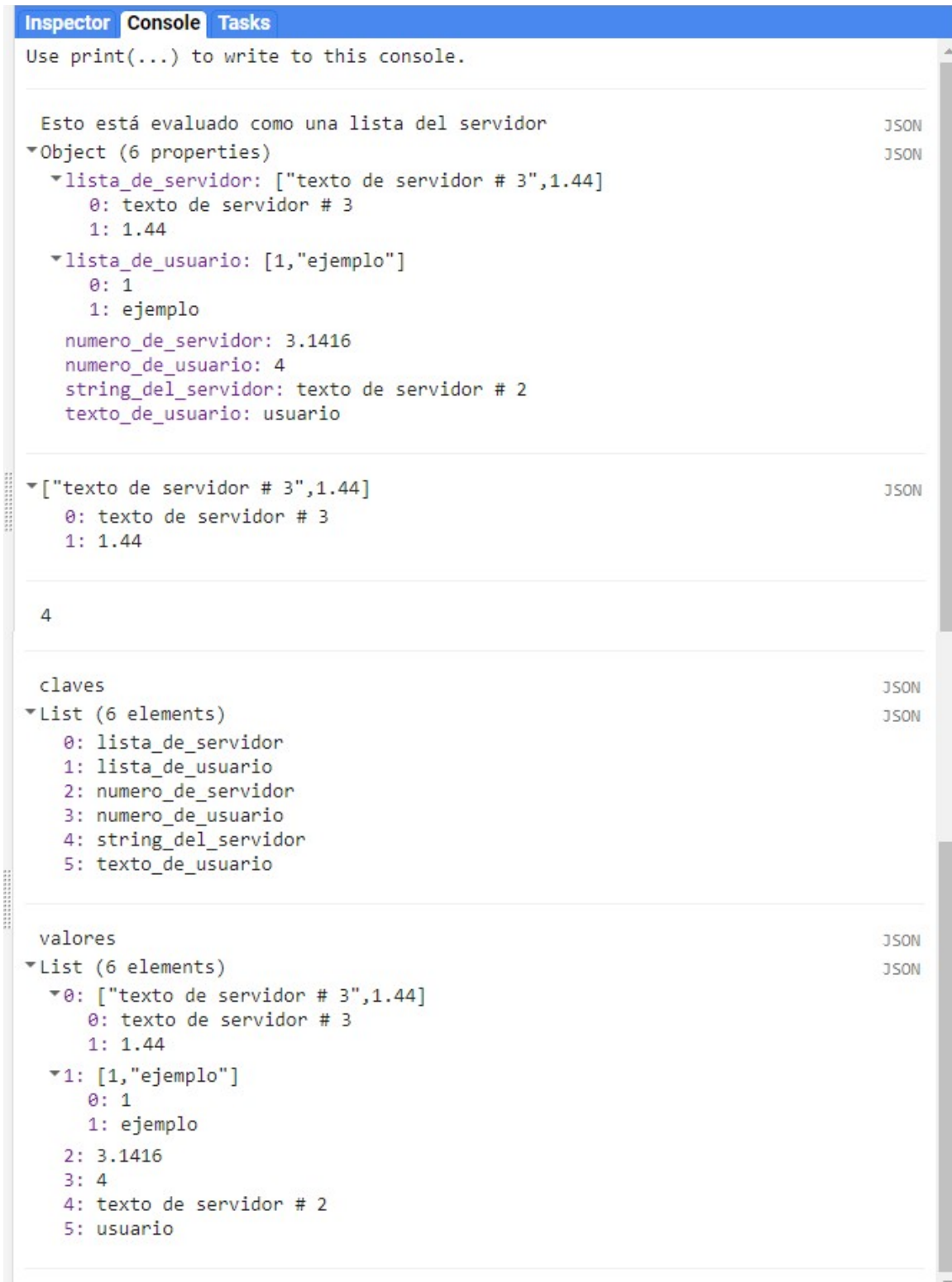
Figura 5.10: Salida de la consola de varios objetos de tipo diccionario del lado del servidor.
