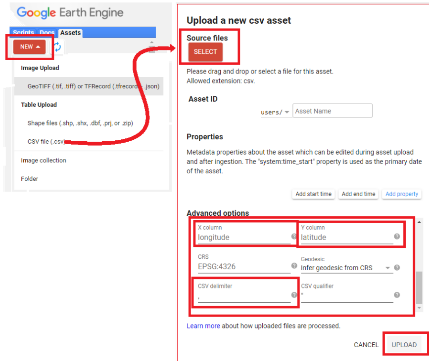
Figura 4.1b: Opciones disponibles para importar datos tipo CSV, especificar (si existe) columna de longitud y latitud (solo acepta punto decimal), y tipo de delimitador.
