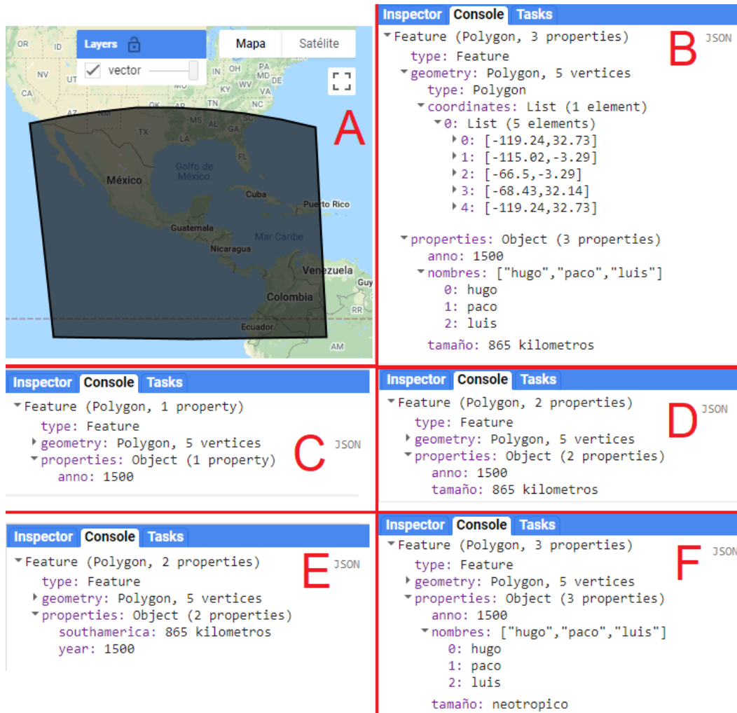
Figura 7.1: Visualización del vector (A). La salidas de la consola mostrando el vector creado con coordenadas y propiedades (B). La selección (ejercicio10.1) de una propiedad (C); de dos propiedades (D); renombrar esas propiedades (E) y reescribir propiedades (ejercicio 10.2) (F)..
